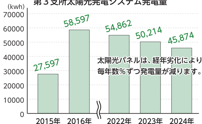
第3支所太陽光発電システム発電量
